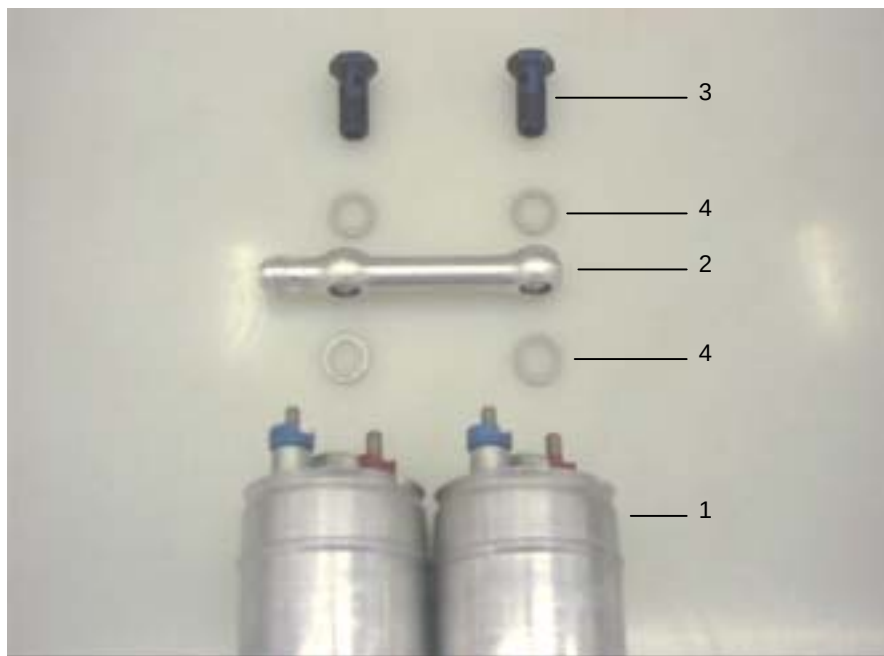
Kraftstoffpumpeneinheit
